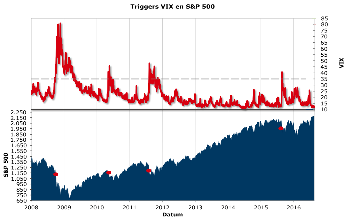
Figuur 2 – Verloop VIX en S&P 500 van 2008
